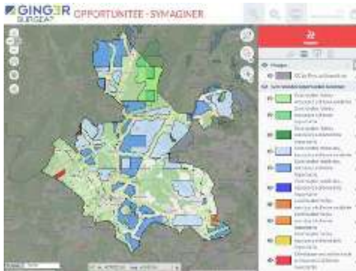
Figure 42 : Traduction du gisement en nombre de mâts installables – Source : OPPORTUNITEE BURGEAP
