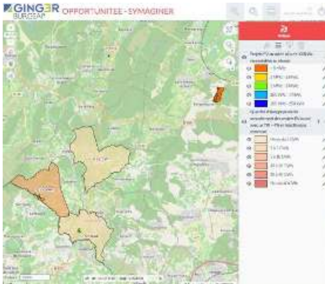
Figure 39 : Synthèse du gisement solaire photovoltaïque au sol, sur friche (projets ayant un TRI supérieur à 4%) en GWh – Source : OPPORTUNITÉ BURGEAP
