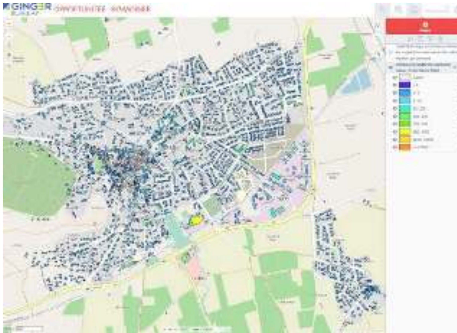
Figure 16 : Gisement solaire photovoltaïque sur ombrière, en injection (projets ayant un TRI supérieur à 4%) en MWc installables, Calvisson– Source : OPPORTUNITÉ BURGEAP
