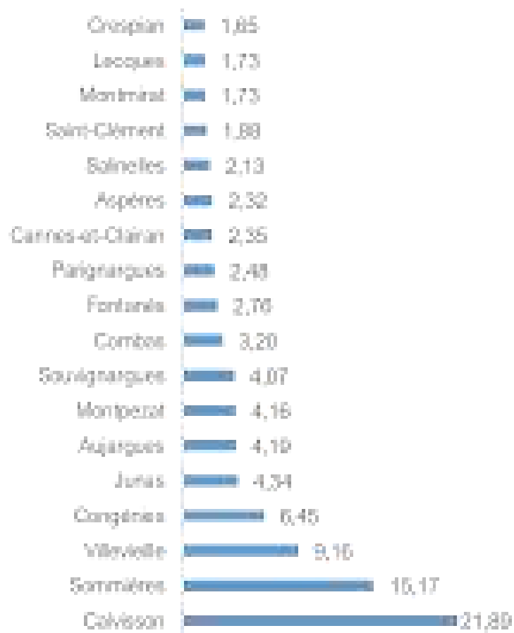
Figure 15 : Synthèse du gisement solaire photovoltaïque sur toiture, en injection (projets ayant un TRI supérieur à 4%) en GWh par an, par commune – Source : OPPORTUNITEE BURGEAP
