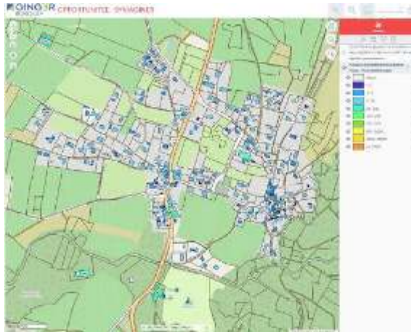
Figure 33 : Gisement solaire photovoltaïque sur ombrière, en injection (projets ayant un TRI supérieur à 4%) en MWc installables, Crespian – Source : OPPORTUNITEE BURGEAP
