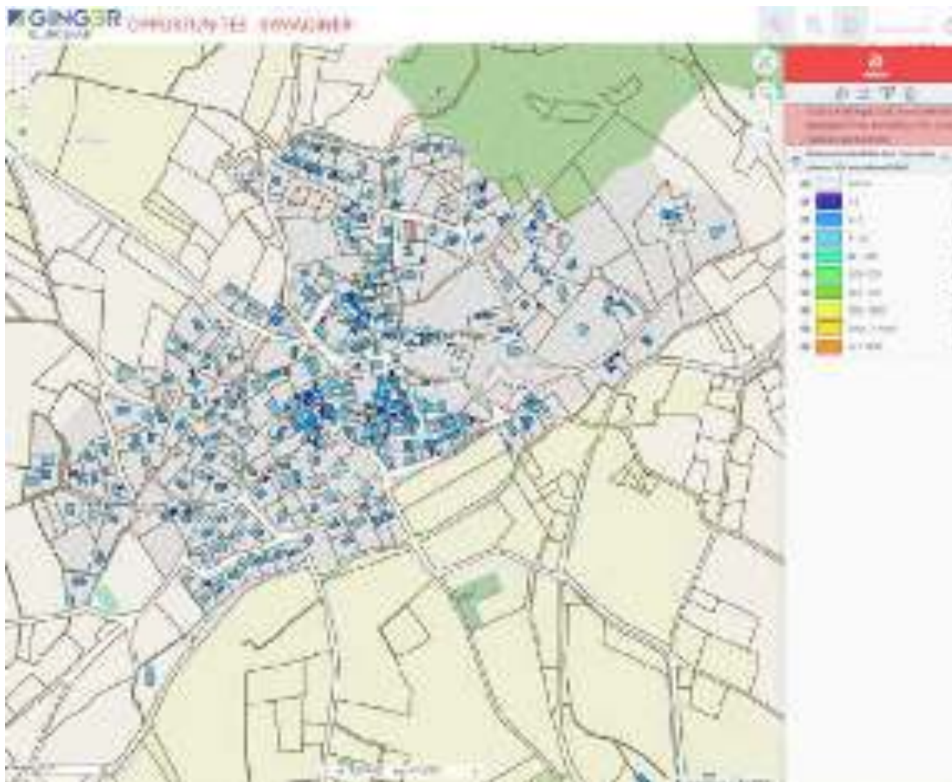
Figure 26 : Gisement solaire photovoltaïque sur ombrière, en injection (projets ayant un TRI supérieur à 4%) en MWc installables, Parignargues – Source : OPPORTUNITEE BURGEAP
